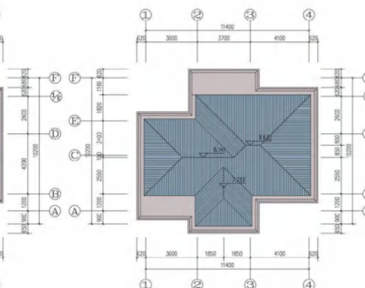
屋顶平面图
