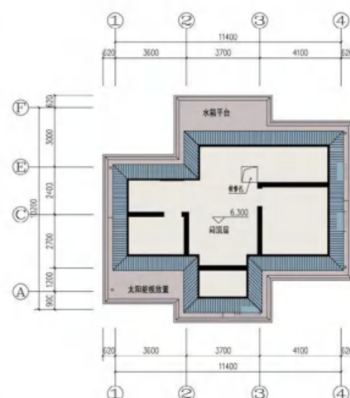
屋顶平面图
