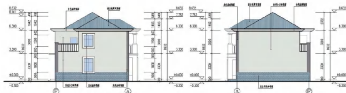
⑦~④轴立面图
