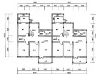
一层平面图 1:100
