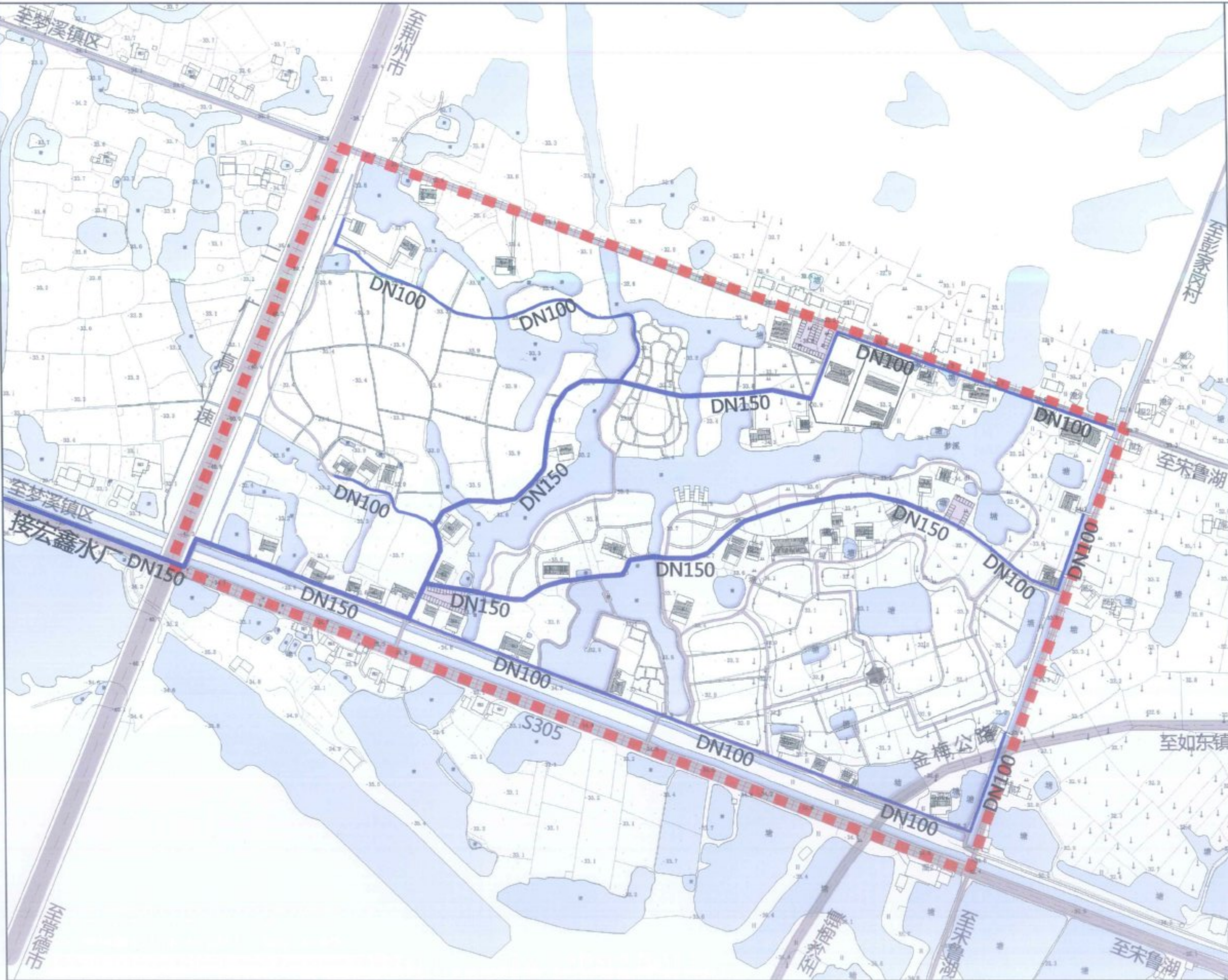
17 居民点给水工程规划图
