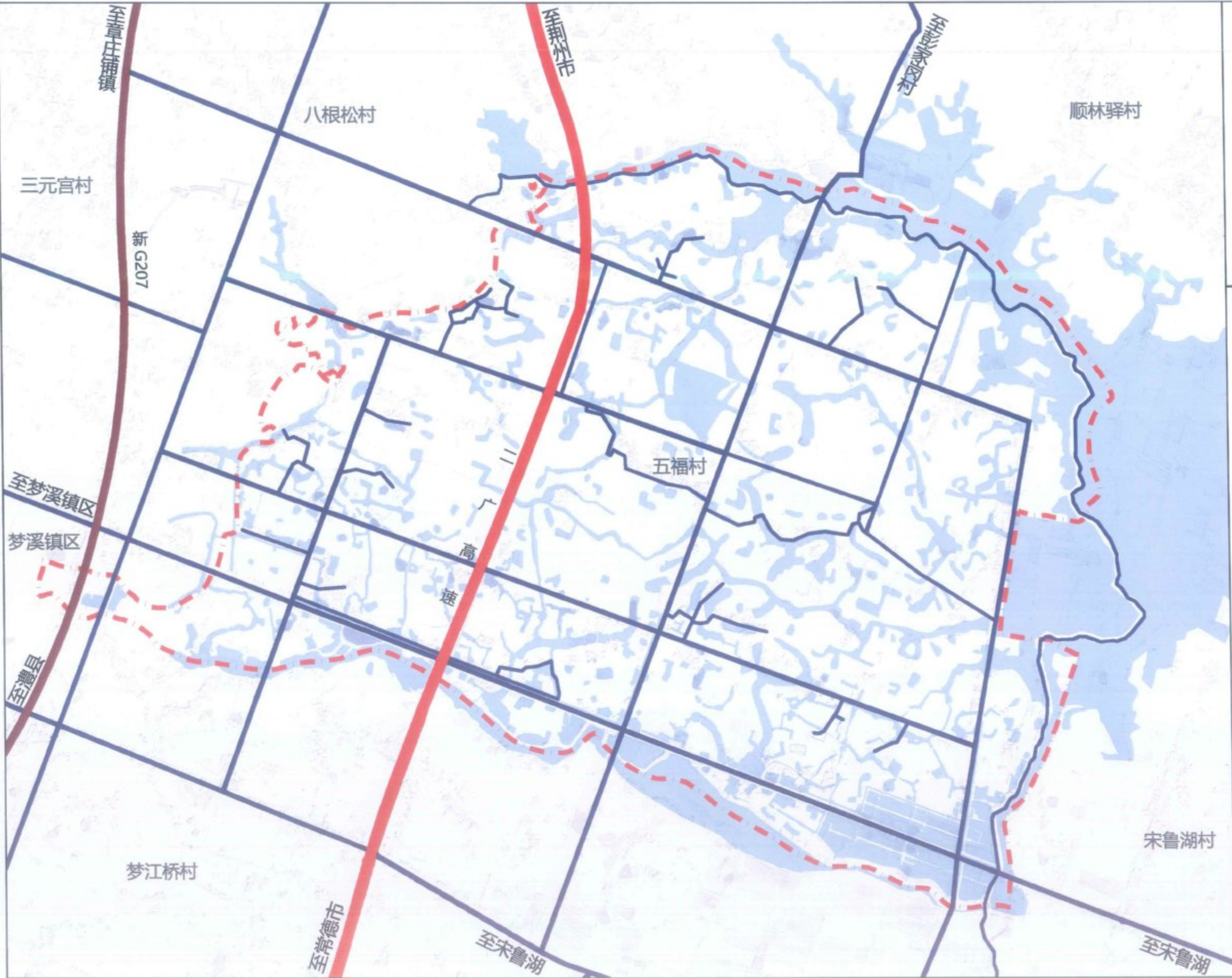
03 村域道路交通现状图
