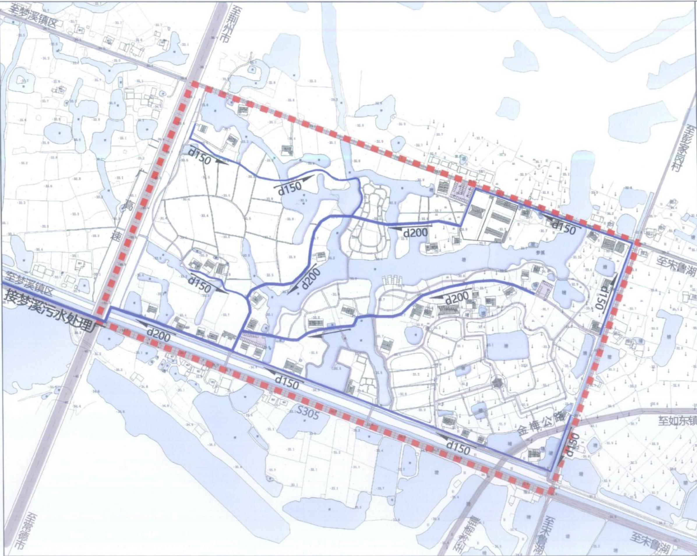
18 居民点污水工程规划图
