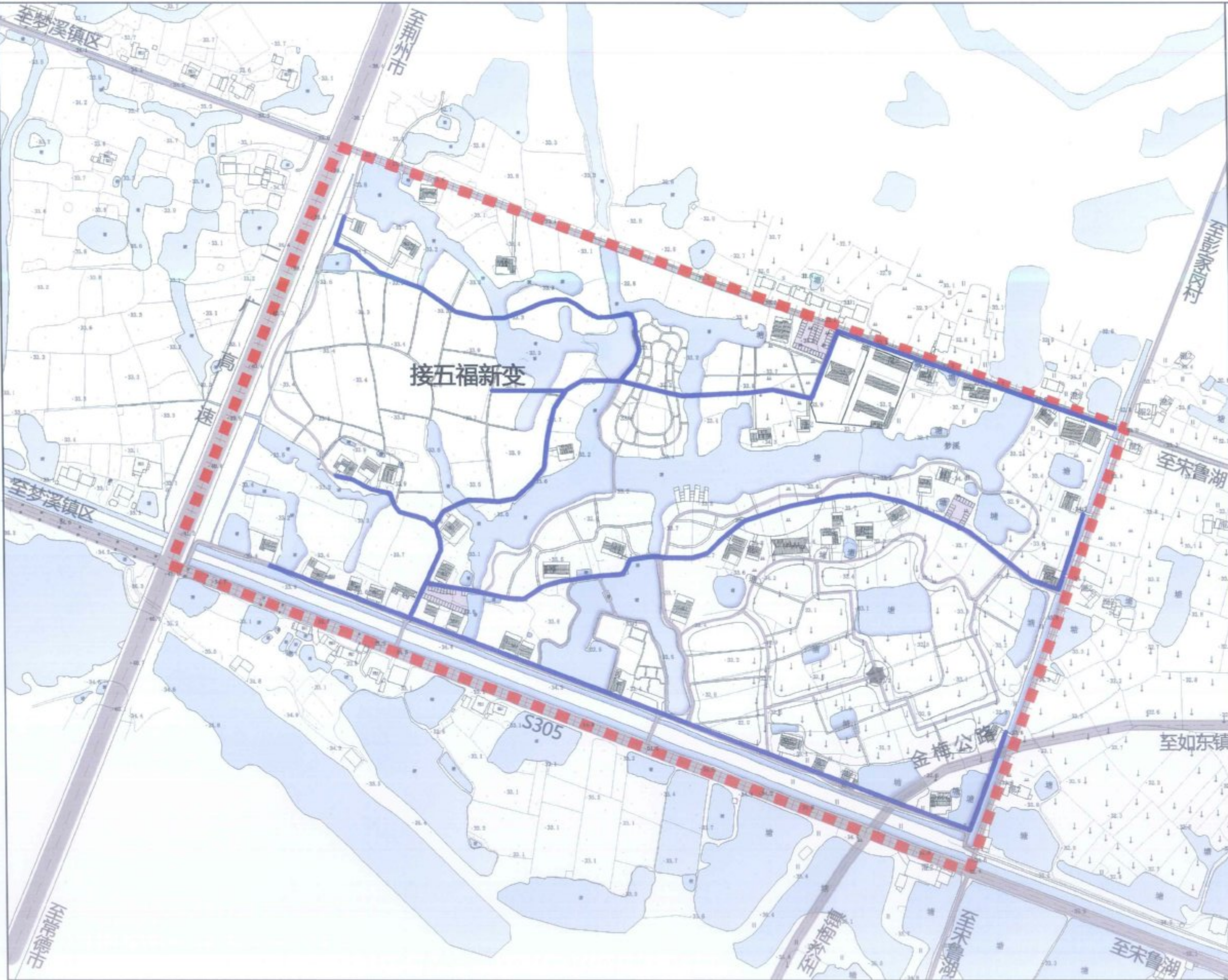
19 居民点电力工程规划图
