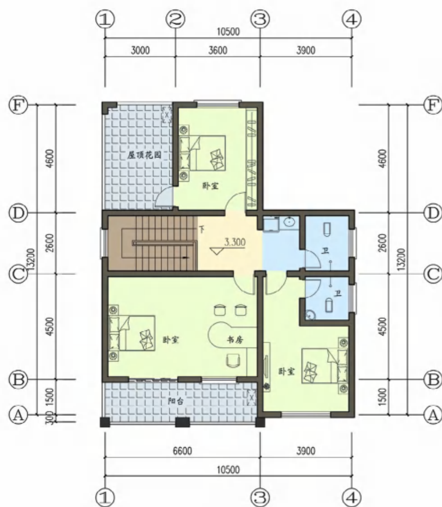
二层平面图
