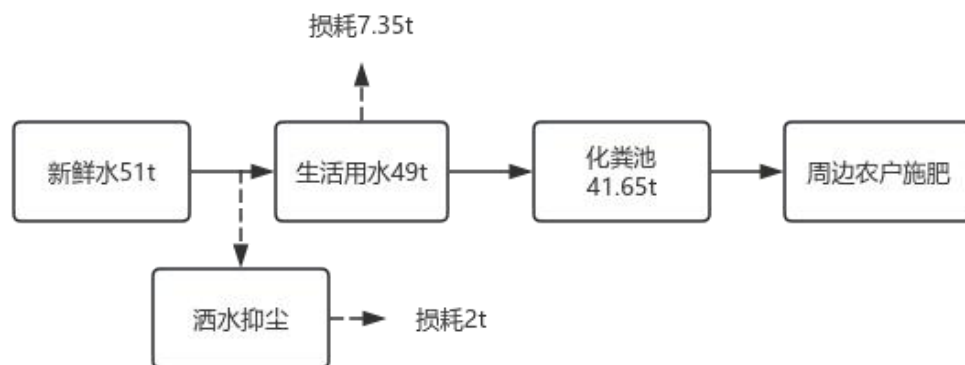
图 2-1 水平衡图
