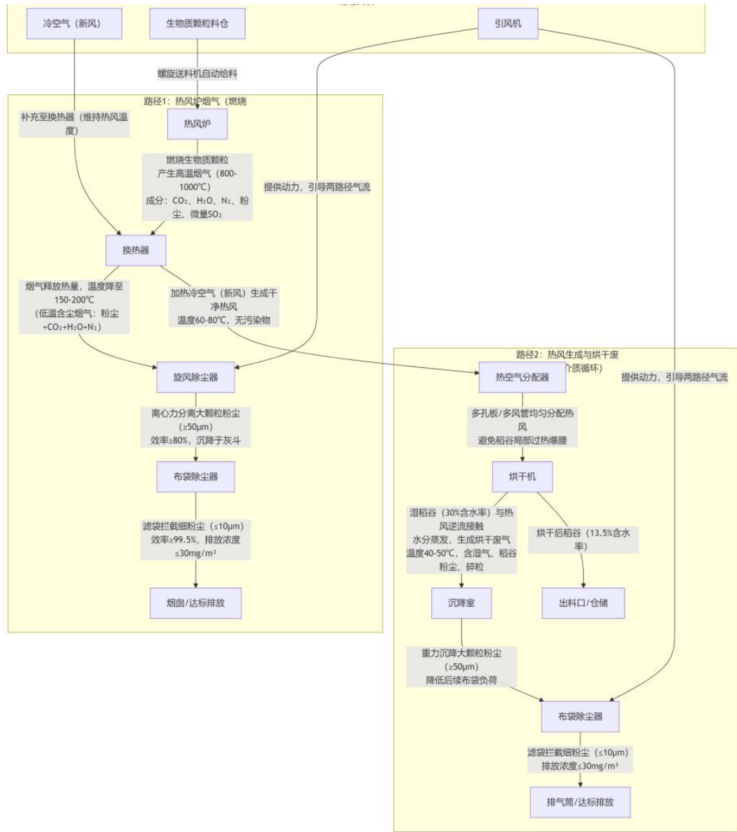
图 2-4 热风炉烟气、热风+烘干废气的走向图
