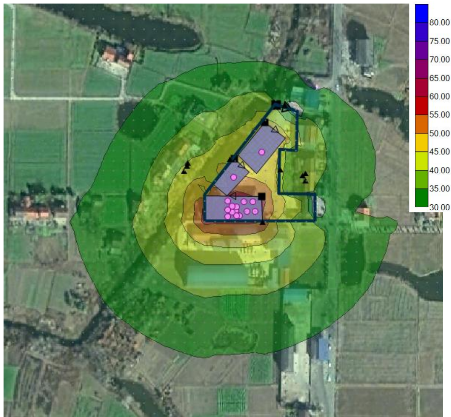
图 4-1 昼间噪声预测等声级线图
