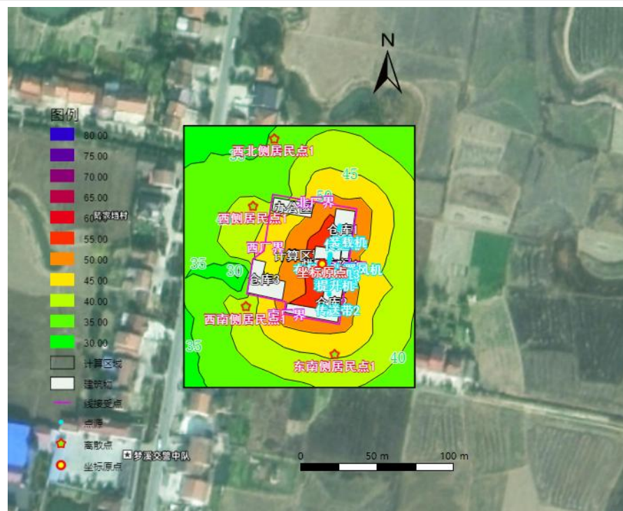
图 4.3-4 昼间噪声贡献值等声级线图
