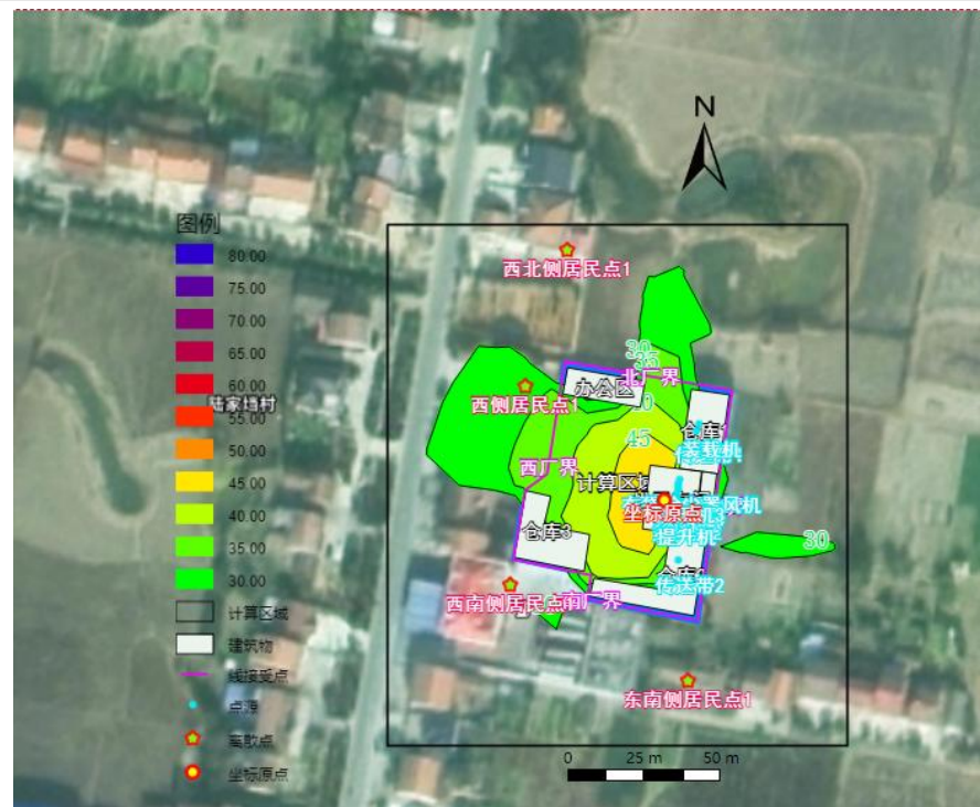
图 4.3-5 夜间噪声贡献值等声级线图
