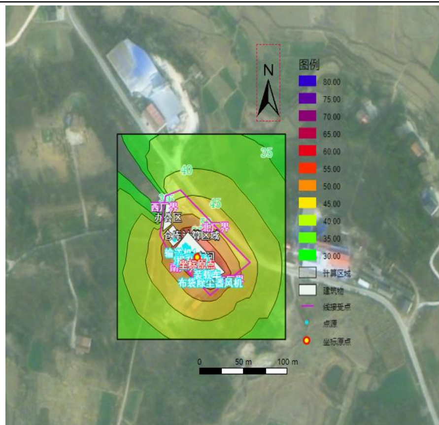
图 4.3-4 昼间噪声贡献值等声级线图
