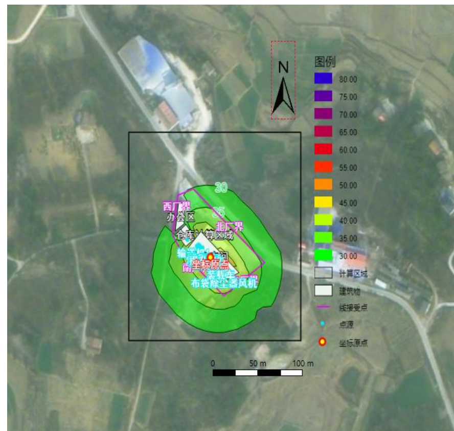
图 4.3-5 夜间噪声贡献值等声级线图
