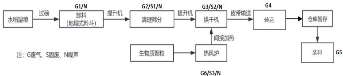
图 2-4 工艺流程及产污环节图
