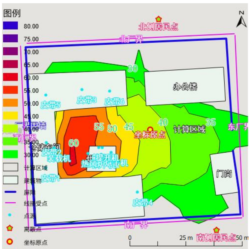
图 4.3-3 夜间噪声贡献值等声级线图
