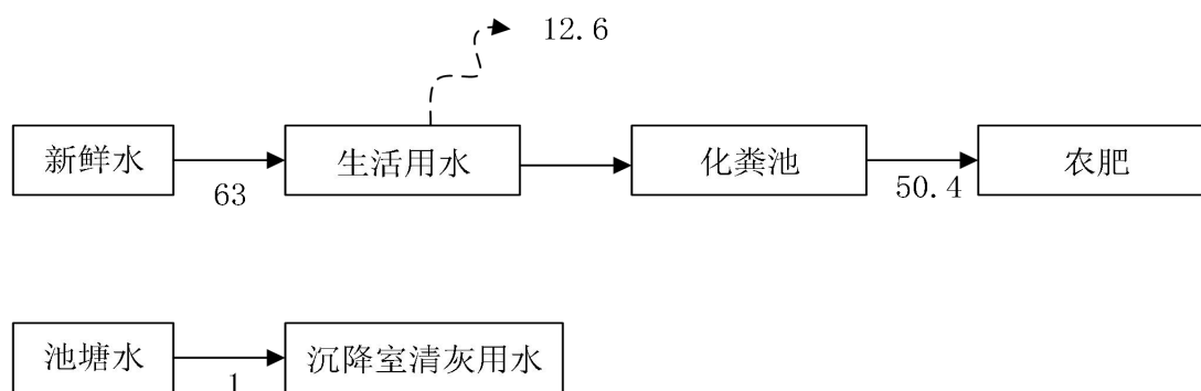
图 2-1 项目用水平衡图（m 3 /a）
