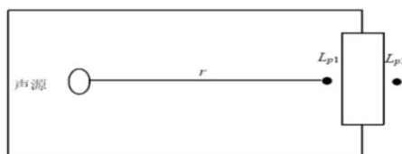
图 4.3-1 室内声源等效为室外声源图例
