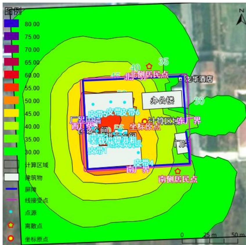
图 4.3-2 昼间噪声贡献值等声级线图
