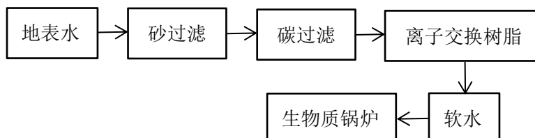
图 2-3 软水制备工艺流程
