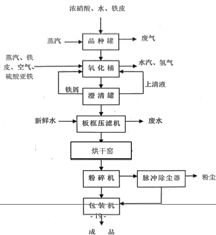
图 2-4 原有工艺流程及产污环节图（硫酸盐湿法氧化铁红）
