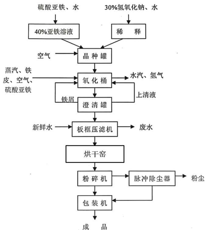
图 2-5 原有工艺流程及产污环节图（硫酸盐湿法氧化铁黄）
