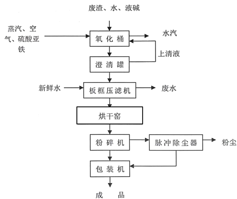
图 2-6 原有工艺流程及产污环节图（加成法氧化铁黑）
